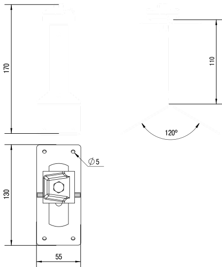
Рисунок 1 – Габаритные размеры
