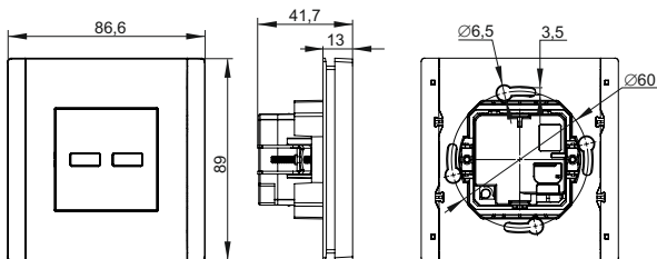
g) Розетка / socket / prizele / занггуп / rozetkalari USB A+A
