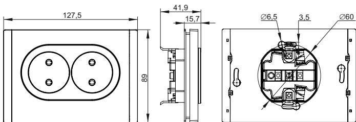
h) Розетка двухместная без контактов заземления / Double socket without grounding contacts / Жерге туйықтау түйіспелерінсіз екі орынды розетка / Priză dublă fără contacte de împământare / Газардуулалт контактгүй давхар залгуурууд / Yerga ulanish kontaktlari mavjud bo'lmagan ikki o'rinli rozetka
