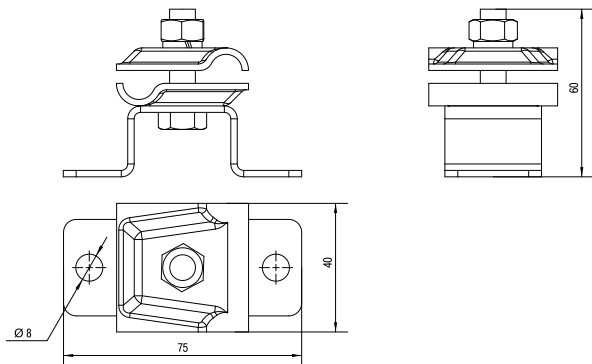
Рисунок 1 – Габаритные размеры
