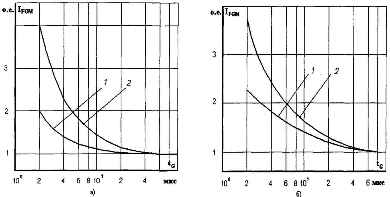
Рис. 2. 14. Зависимость отпирющего импульсного тока управления I_{FGM} от длительности управляющего импульса t_G при температуре перехода T_j = 25 °С (1) и минимально допустимой температуре T_{jmin} (2), U_D = 12 В
