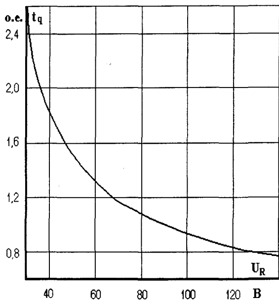
Рис. 2. 8. Зависимость времени выключения t_q от обратного напряжения U_R при максимальной температуре перехода T_{jm} = 125 \text{ }^\circ\text{C} , I_{TM} = I_{T(AV)} , di_T/dt = 5 \text{ А/мкс} , dU_D/dt = 50 \text{ В/мкс} , U_D = 0,67U_{DRM}
