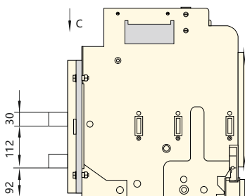
NA8G-6300(I n =6300A) выдвижное исполнение, заднее присоединение, горизонтальные контактные пластины
