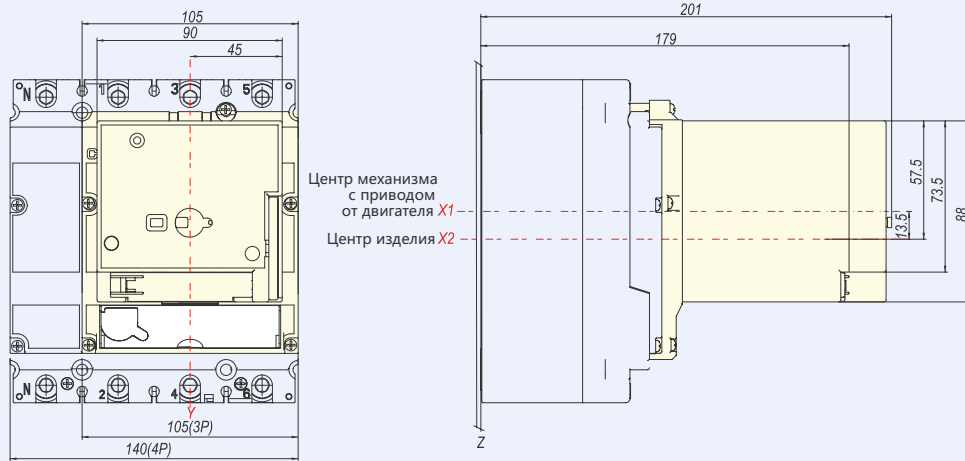
Установочные размеры MOD22-M8
