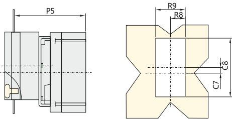
Разметка панели ( для выключателей стационарного и втычного исполнений )
