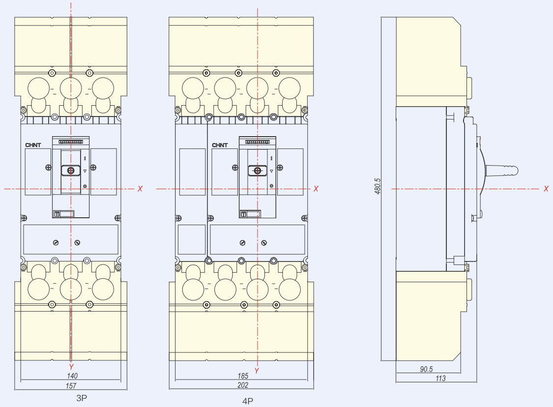
NM8N-400/630, короткая крышка для клемм
