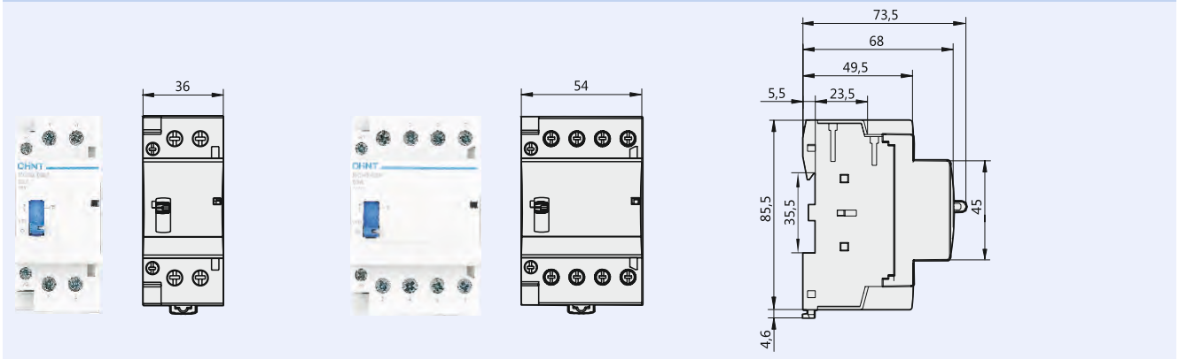
Рисунок 3. NCH8-32M, NCH8-40M, NCH8-63M
