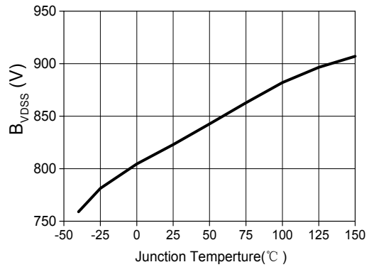
(b) BV_{DS} vs T_j
