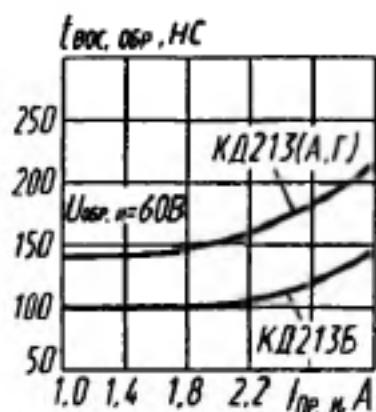
Зависимости времени обратного восстановления от тока
