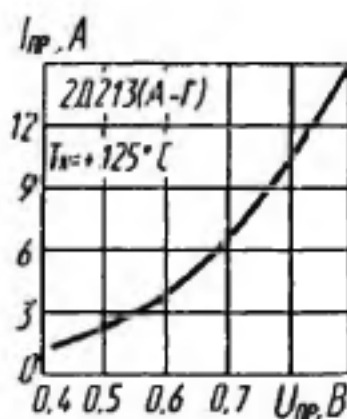
Зависимость прямого тока от напряжения
