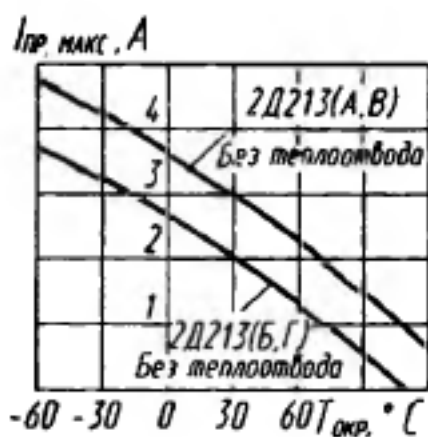
Зависимости допустимого прямого тока от температуры
