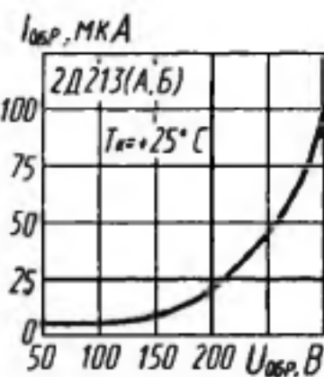
Зависимость обратного тока от напряжения
