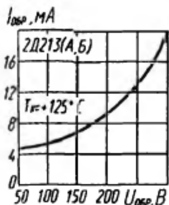
Зависимость обратного тока от напряжения
