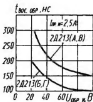
Зависимости времени обратного восстановления от напряжения
