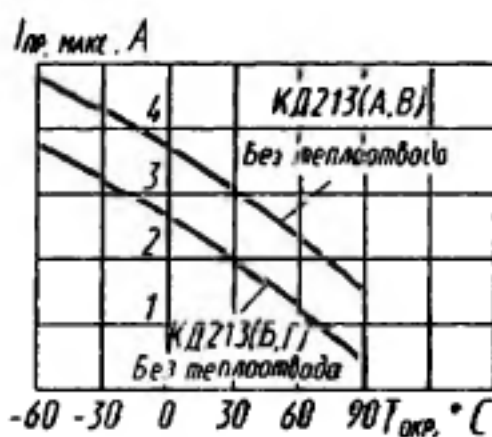
Зависимости допустимого прямого тока от температуры
