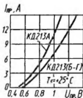
Зависимость прямого тока от напряжения
