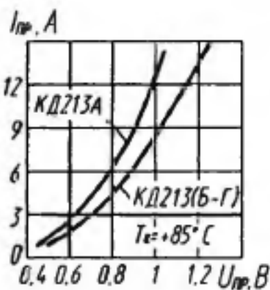
Зависимость прямого тока от напряжения
