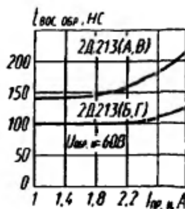
Зависимости времени обратного восстановления от тока
