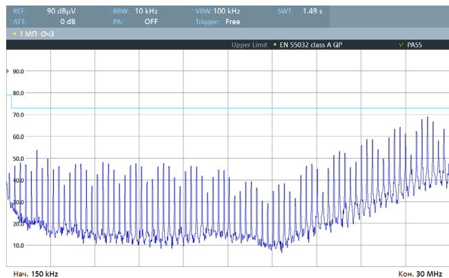
Рис. 37. Спектрограмма работы VDRI20B24 по схеме включения [Рис. 3], измерения произведены в соответствии с EN 55032 Class A (0,15–30 МГц).
