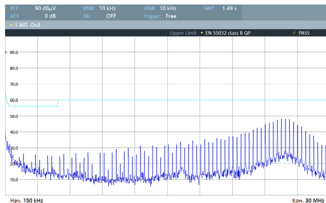
Рис. 36. Спектрограмма работы VDRI20B05 по схеме включения [Рис. 4], измерения произведены в соответствии с EN 55032 Class B (0,15–30 МГц).
