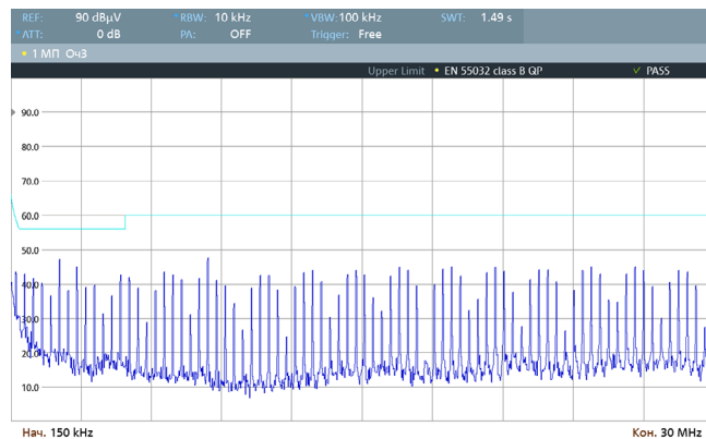
Рис. 38. Спектрограмма работы VDRI20B24 по схеме включения [Рис. 4], измерения произведены в соответствии с EN 55032 Class B (0,15–30 МГц).
