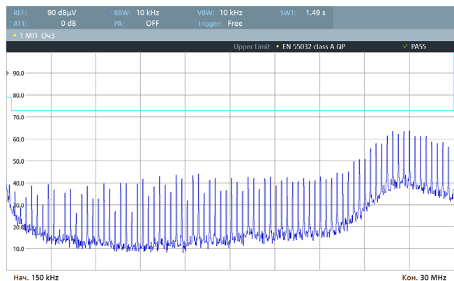
Рис. 35. Спектрограмма работы VDRI20B05 по схеме включения [Рис. 3], измерения произведены в соответствии с EN 55032 Class A (0,15–30 МГц).
