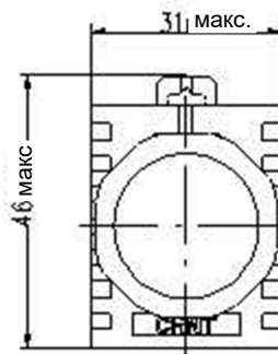
Рис.5 NP8-11XD
