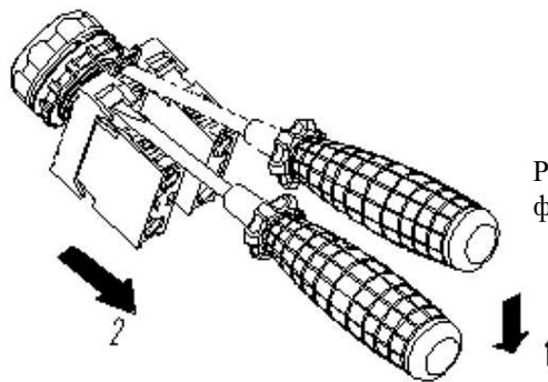
Рис. 10 Процесс установки
