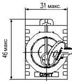
Рис.4 NP8-11MD
