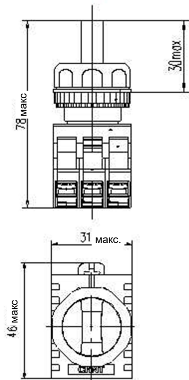
Рис.4 NP8-11XD
