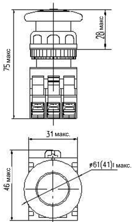
Рис.4 NP8-11MD
