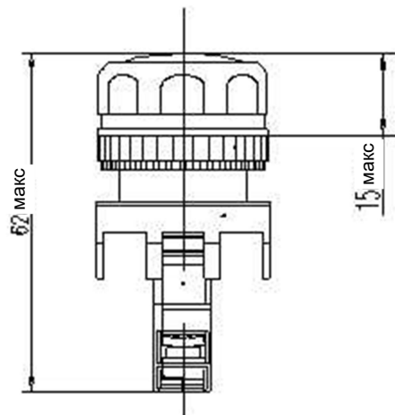
Рис.7 NP8-11ZS
