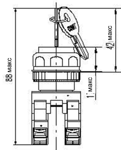
Рис.6 NP8-11SD
