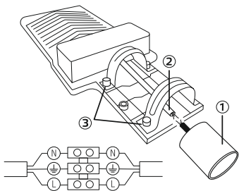
Рис. 1. Монтаж светильника
