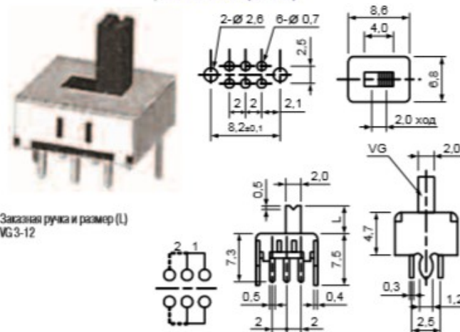
SS22F07(2P2T)
