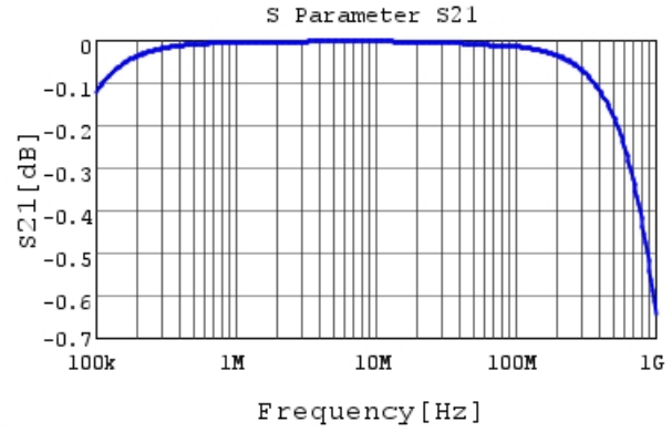
RDER71H104K0K1H03B S21 DC0V, 25degC
