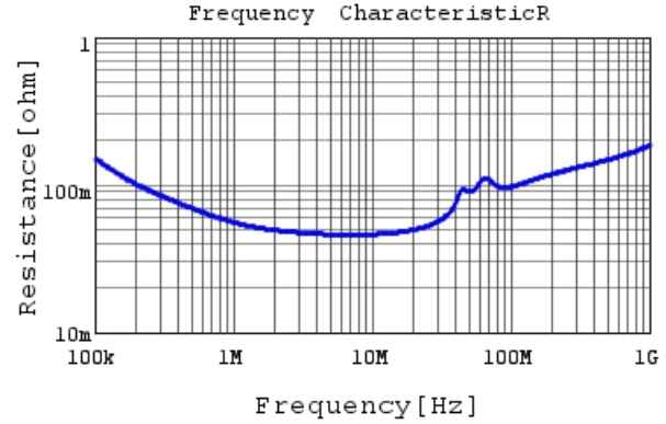
RDER71H104K0K1H03B R DCOV, 25degC
