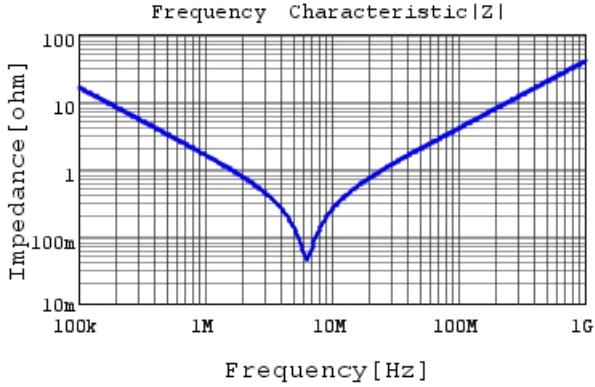
RDER71H104K0K1H03B |Z| DCOV, 25degC
