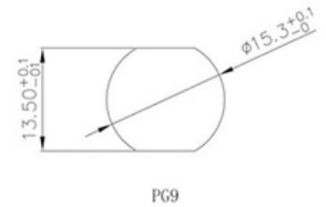
PG9 安装尺寸 Installation dimension
