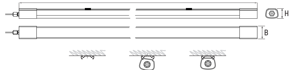
Рис.2 Габаритные размеры светильников
