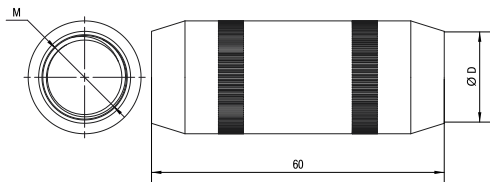
Рисунок 1 – Габаритные размеры
