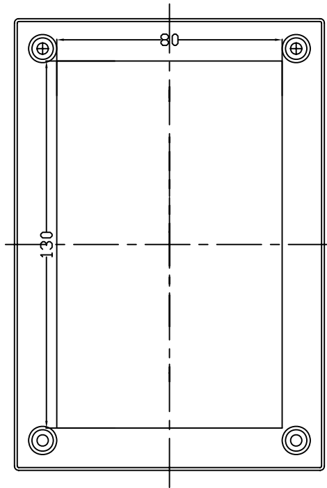
上盖反面图
