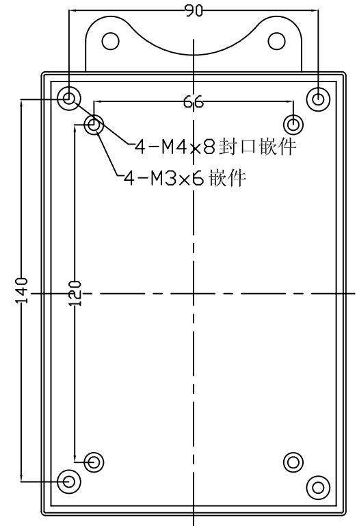
下盖正视图
