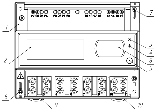
Рисунок 2.2 – Внешний вид и нумерация контактов счетчика счетчика CE307 R33
