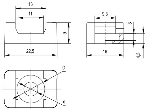
Рисунок 1 – Площадка монтажная ПМ
