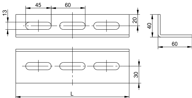
Рисунок 13 – Профиль перфорированный L-образный ГЭМ К242
