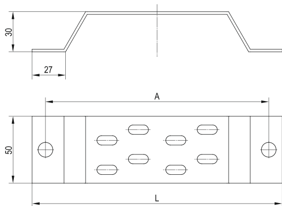
Рисунок 6 – Стойка настенная
