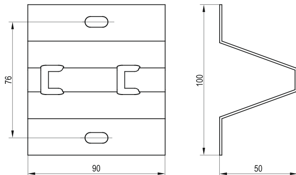
Рисунок 4 – Стойка напольная 100
