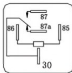
Схемы коммутации
