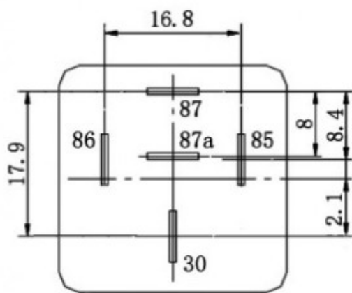
Расположение контактов
