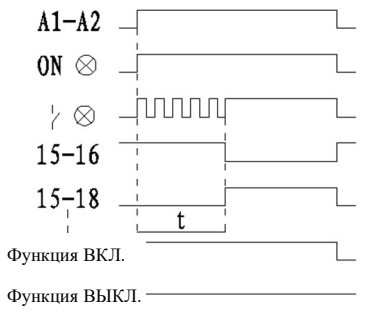
Рис. 19. Диаграмма рабочей последовательности NTE8-M1
