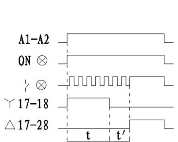
Рис. 18. Диаграмма рабочей последовательности NTE8-Y
