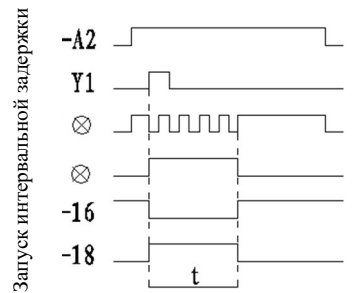
Рис. 26. Диаграмма рабочей последовательности типа В с задержкой времени
