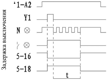
Рис. 22. Диаграмма рабочей последовательности типа С с задержкой времени
