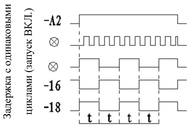
Рис. 24. Диаграмма рабочей последовательности типа Di с задержкой времени
