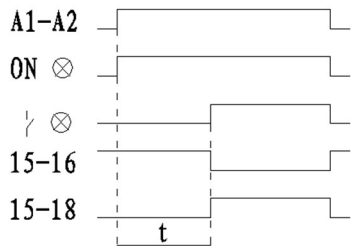
Рис. 15. Диаграмма рабочей последовательности NTE8-B
