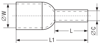
Рис. 2. Наконечники-гильзы втулочные типа Е
