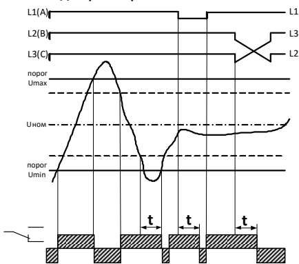
Диаграмма работы РКФ-М05-2-15
