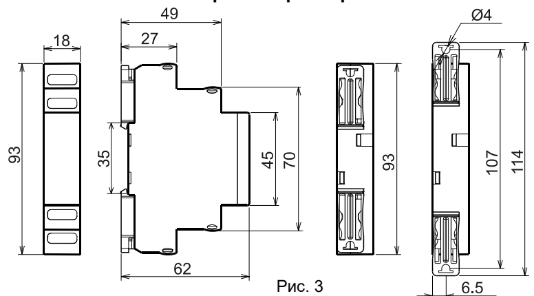
Габаритные размеры
