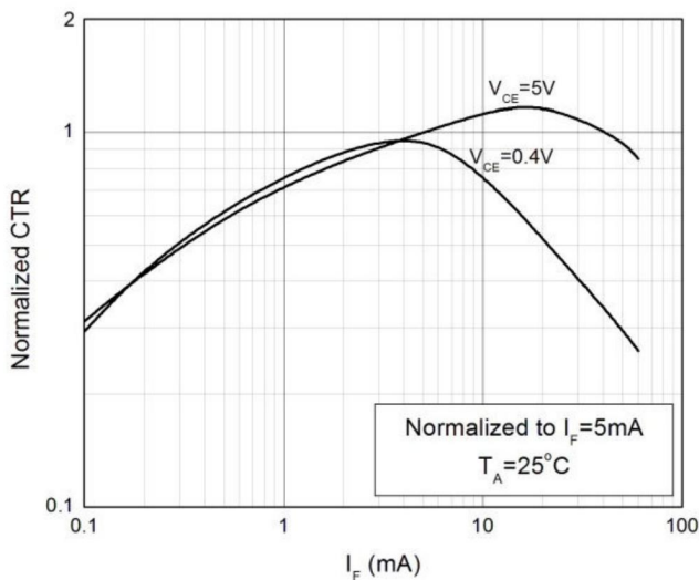
图 4 CTR- I_F 特性曲线
