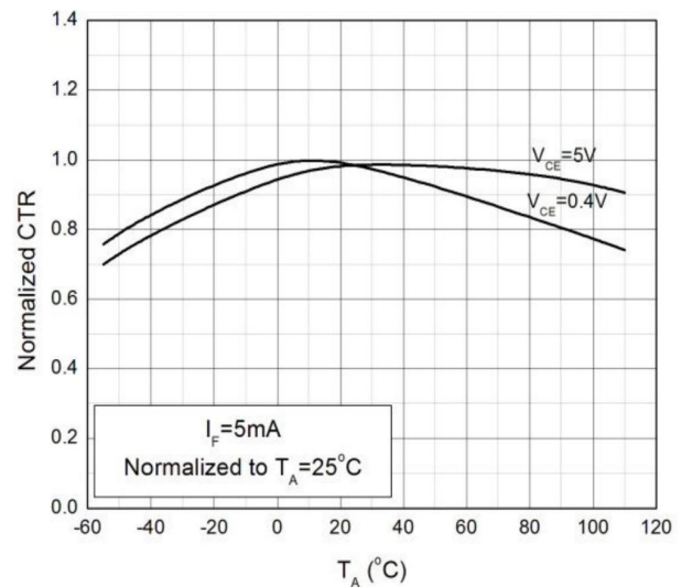
图 5 CTR- T_A 特性曲线
