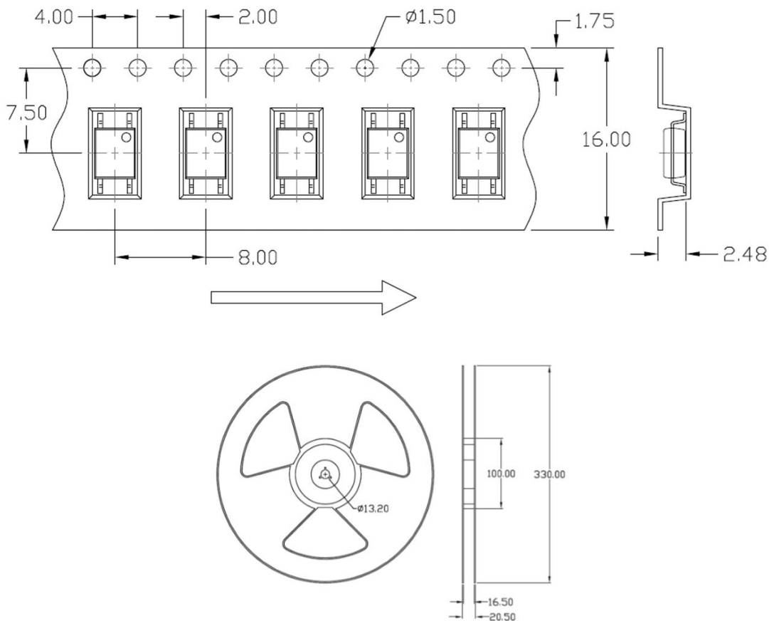
图 9 编带包装示意图
