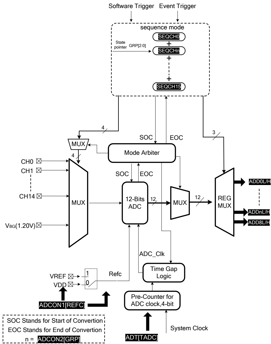
图8.8-1 ADC模块图
