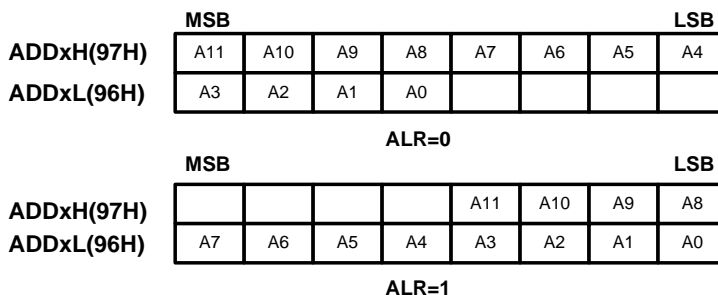
图8.8-3 ADC转换结果存储方式示意图
