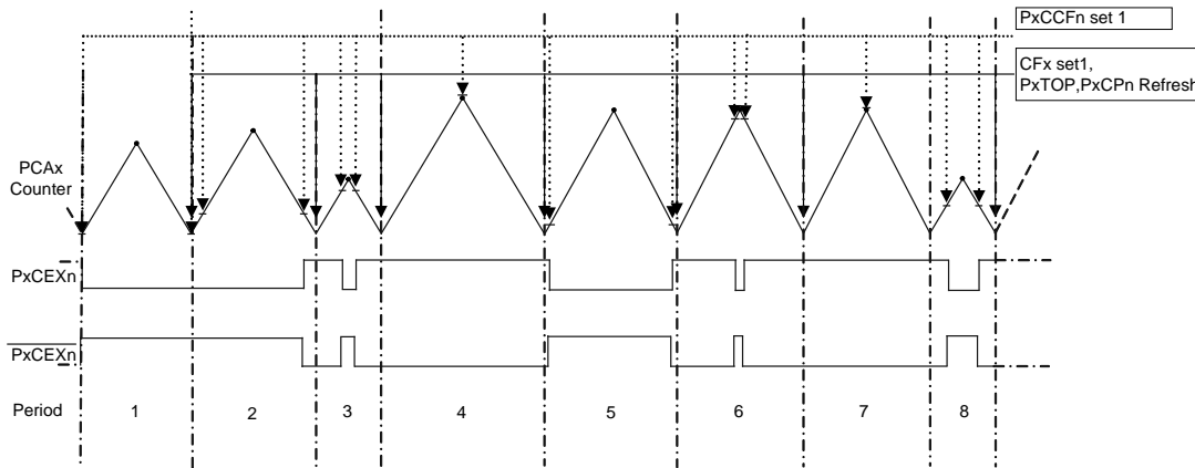
图7.9-15 16位XPPWM波形图
