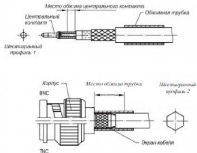
Схема кримпирования разъемов типа BNC/ TNC на коаксиальный кабель
