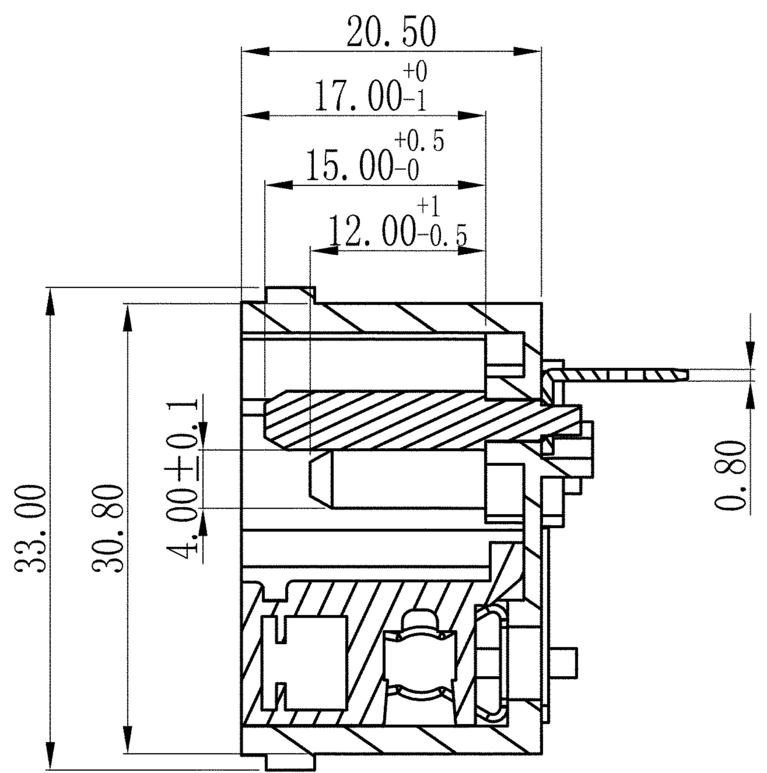
SECTION A-A
