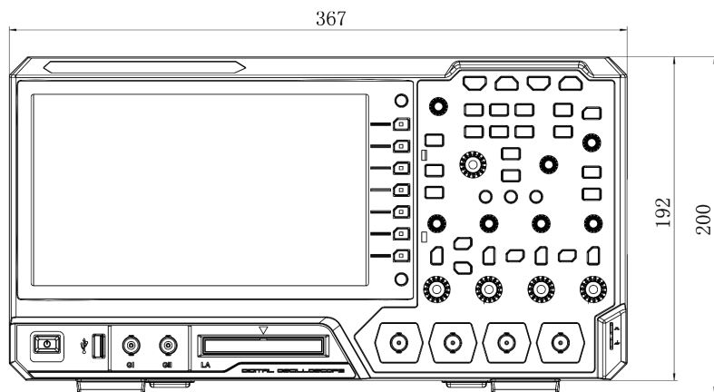
Вид спереди, единица измерения: мм
