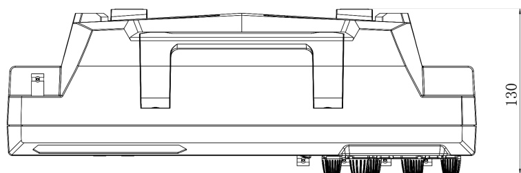
Вид сверху, единица измерения: мм
