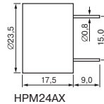
HPM24AX
