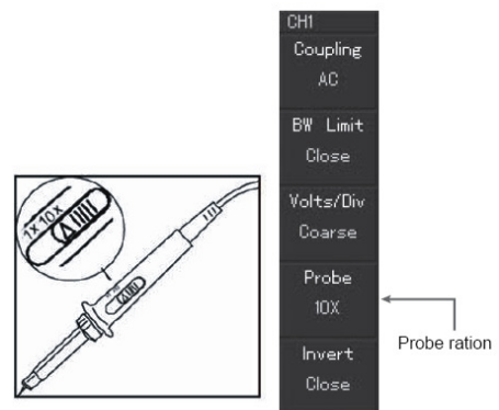
Рисунок 1-6 Установка коэффициента ослабления на щупе осциллографа.
