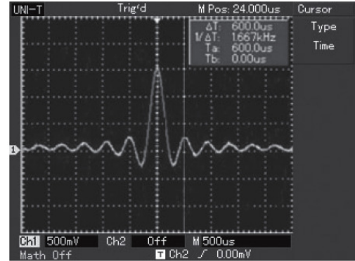
Рисунок 3-6 Курсорное измерение частоты сигнала
