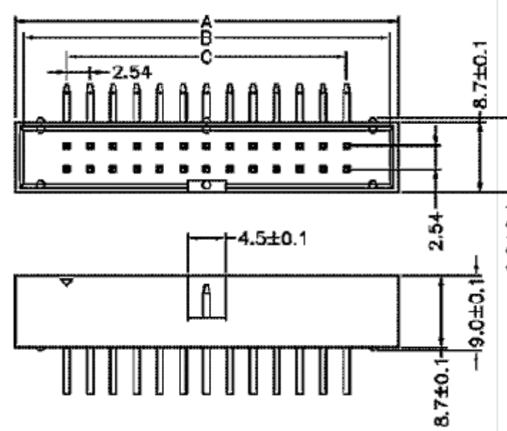
IDC-xxMR - двухрядные вилки на плату угловые
