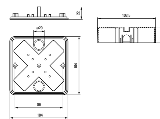
Коробка установочная КМР-030-032 и КМР-030-032kg
