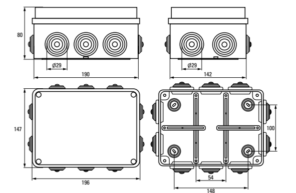
Коробка установочная KMP-050-042
