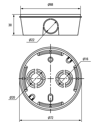
Коробка установочная KMT-195
