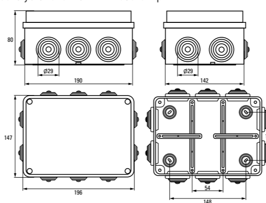
Коробка установочная КМР-050-042рк
