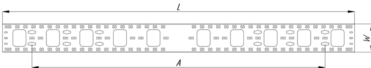
Рисунок 2 – Органайзер кабельный вертикальный 150
